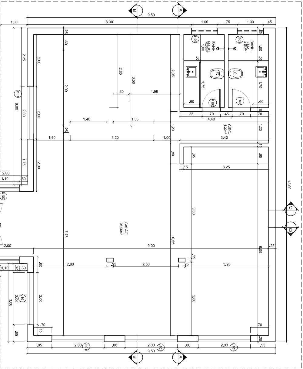
1 PLANTA BAIXA ESCALA: 1/750
